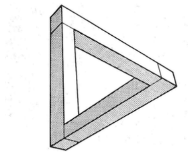
Figura 1.2: Tribarra , R. Penrose.
