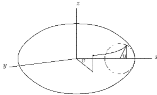
Figura 2.2: Rappresentazione del toro.
