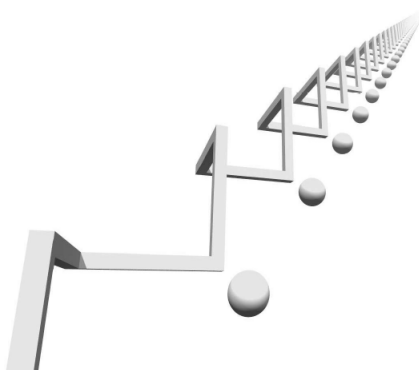
Figura 3.8: Una tribarra e una sfera attraverso una proiezione di rivestimento da \mathbb{R}^3 al 3-cilindro.
