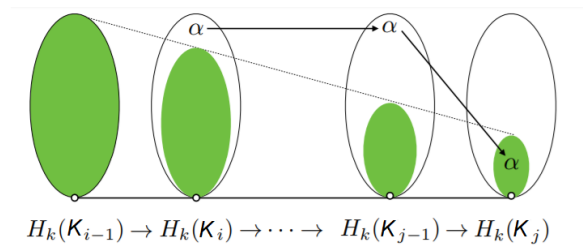
Figura 1.5: La classe di omologia \alpha è nata in K_i poiché non è nell'immagine di i_k^{i-1, i} colorata in verde. Muore in K_j poiché è contenuta nell'immagine della mappa indotta dall'inclusione K_{j-1} \subset K_j ma non nell'immagine della mappa indotta dall'inclusione K_{i-1} \subset K_{j-1}
