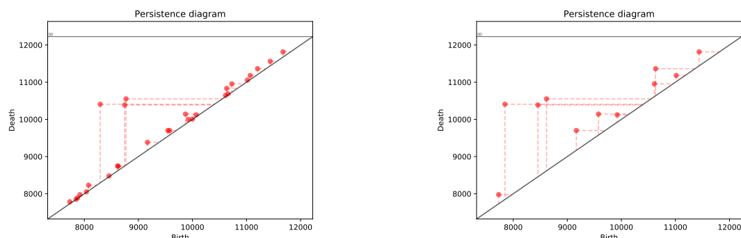
Figura 3.18: Diagrammi di persistenza per steady e ranging hub per (G_1, <, max_-) .
